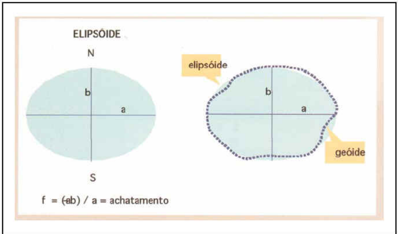
Figura 4. Representação do elipsóide e do geóide.
